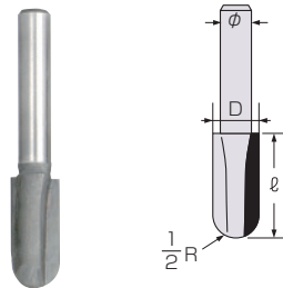
トリマーサジ面ビット Trimmer Spoon-Shaped Surfaces
