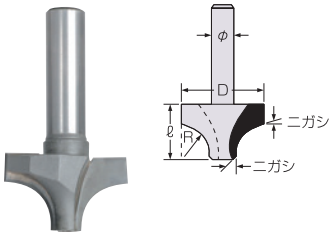
ボーズ面ビット Quarter Rounded
