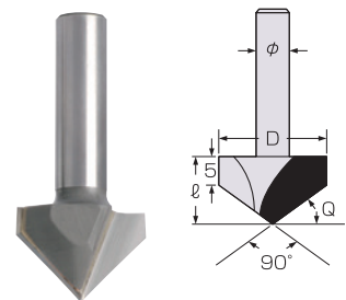
V溝ビット V-Shaped Grooving
