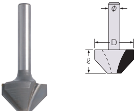
トリマーカク面ビット Trimmer Square
