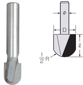
U溝ルータービット U-Shaped Grooving
