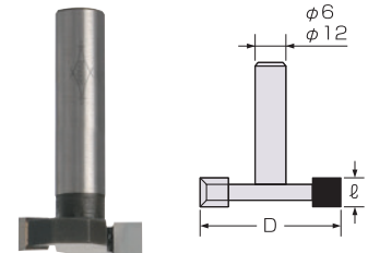
横溝ビット Side Grooving
