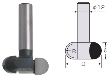
出丸ビット Lobe Rounding
