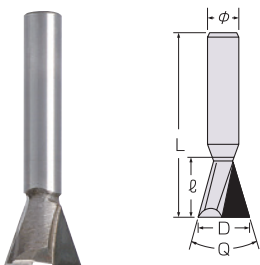
アリ溝ビット Dovetail Grooving
